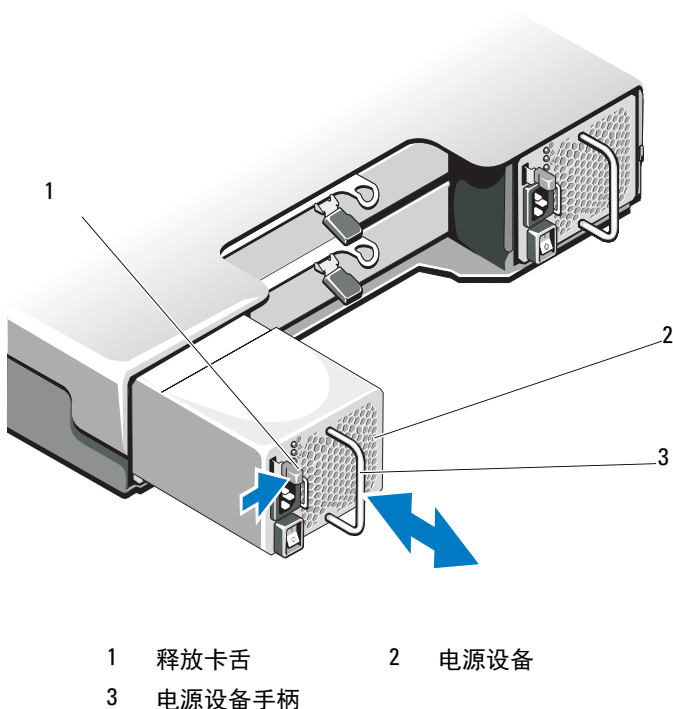
图 16-11. 卸下和安装电源设备 / 冷却风扇模块
